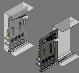
Wandauszüge Wall drawers
