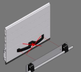
Umrüstsatz R-5001-FR/S Converting Unit R-5001-FR/S
